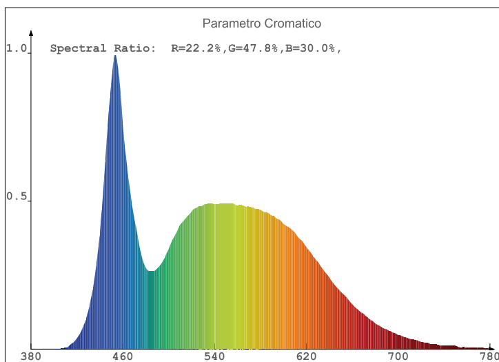
Diagrama de Distribución Luminica
