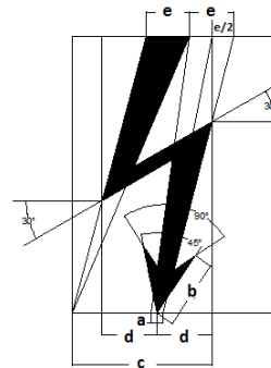
Figura 6.1. Símbolo de riesgo eléctrico
