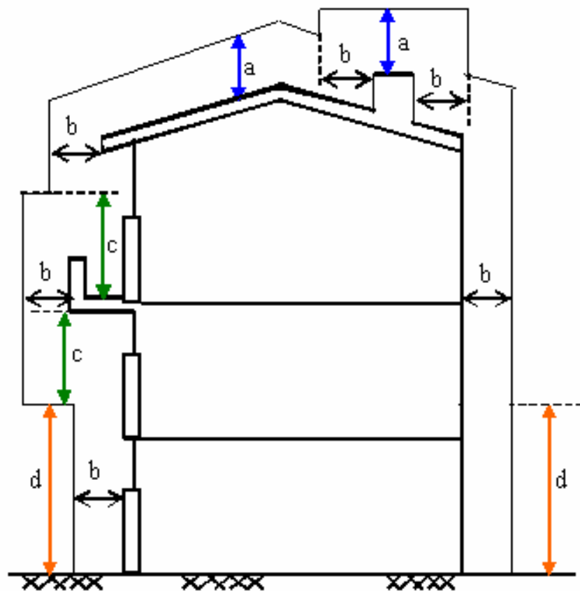
Figura 5. Distancias de seguridad en zonas con construcciones
