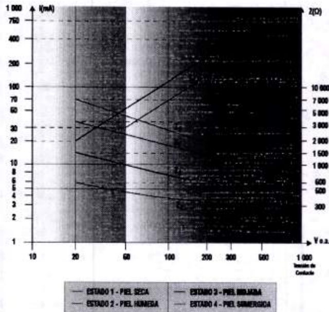
Figura 1.5.1.2. b. Impedancia del cuerpo.
