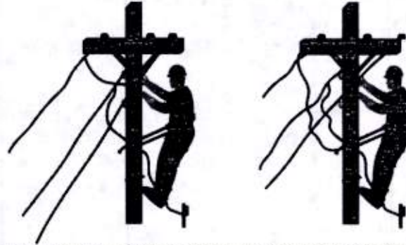
Figura 3.17.25. a. Montajes típicos de puestas a tierra temporales en redes aéreas. Fuente: Adaptada de la Resolución 90708 del 2013.
