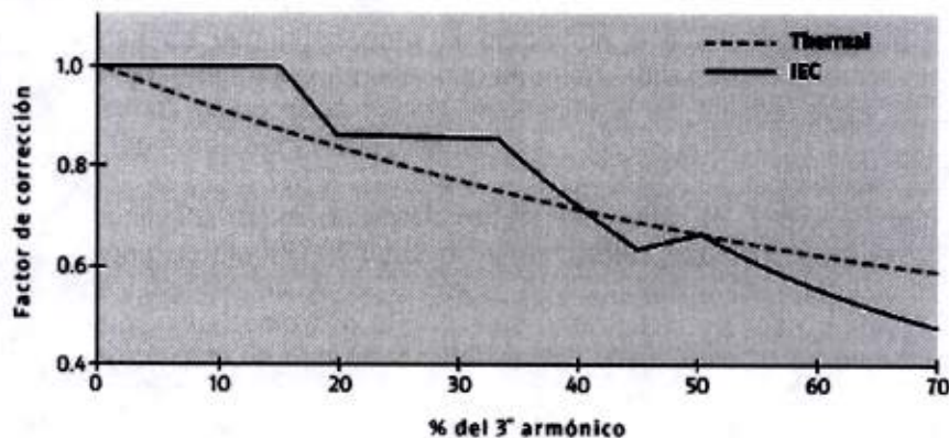
Figura 3.3.3.6. a. Factor de Corrección en función de la proporción de armónicos. Fuente: Adoptada de la norma IEC 60364-5-52.
