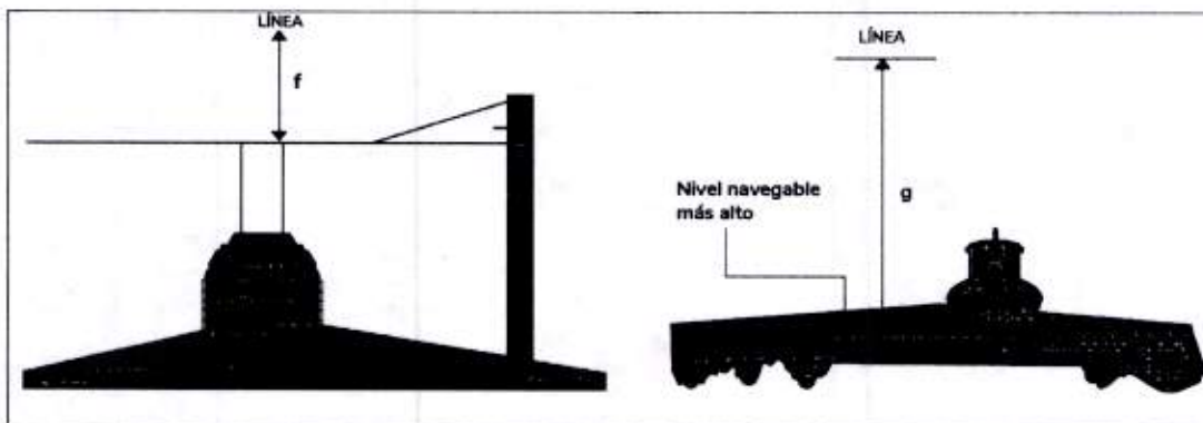
Figura 3.10.2. c. Distancia "f" y "g" para cruces con ferrocarriles y ríos.
