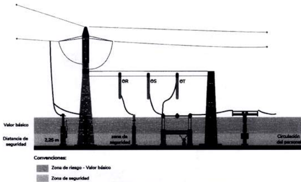
Figura 3.22.1. b. Zona de seguridad para circulación de personal. Fuente: Adaptada de la Resolución 90708 del 2013.
