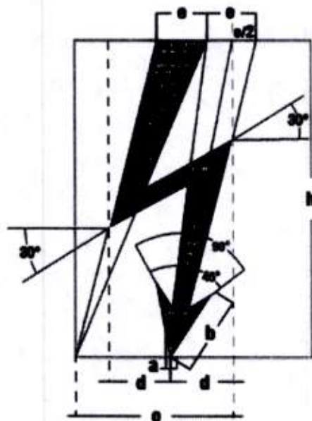
Figura 1.3.3.2. a. Símbolo de riesgo eléctrico. Fuente: Adaptada de la norma IEC 60417.
