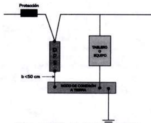
Figura 3.17.14. a. Montaje típico de DPS. Fuente: Adaptada de la Resolución 90708 del 2013.
