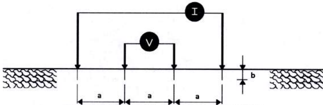
Figura 3.12.4.1. a. Esquema de medición de resistividad aparente. Fuente: Adaptada de la Resolución 90708 del 2013.
