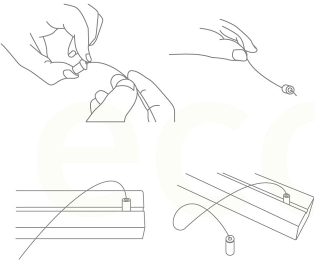
1. Instalación suspendida
